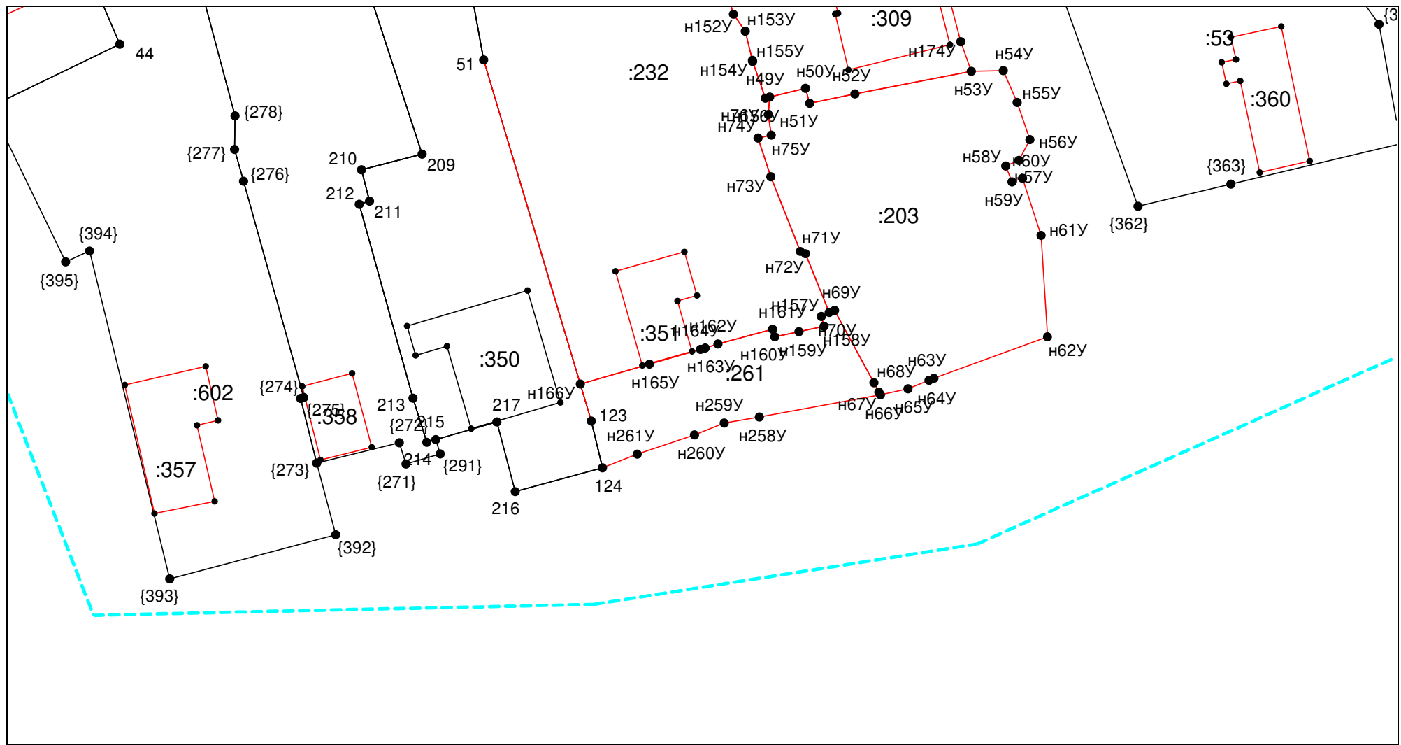
Выносной лист №9
